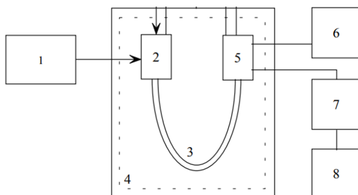
Рис. 4.1. Схема газового хроматографа:
