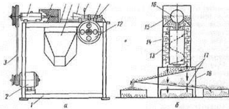
Рис. 61. Агрегат-семеотделитель АС-0,5: а — станок для выверливания стержней шпихи, б — машина для изготовления семян МНС-1; 1 — рама, 2 — электродвигатель, 3 — клиноремная передача, 4 — ось, 5 — стержень, 6 — центрирование, 7 — лопатка, 8 — конус зажимной, 9 — рукоятка, 10 — каретка подвешивания, 11 — упор, 12 — микровыключатель, 13 — барабан вращательный подвешивания, 14 — бункер загрузки, 15 — бункер загрузки, 16 — редуктор, 17 — лоток, 18 — станина.
