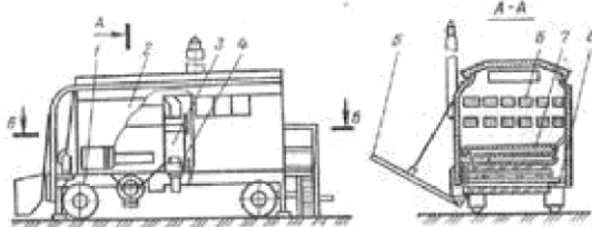
Рис. 59. Шинкосушилка передвижная ШП-0,06:
